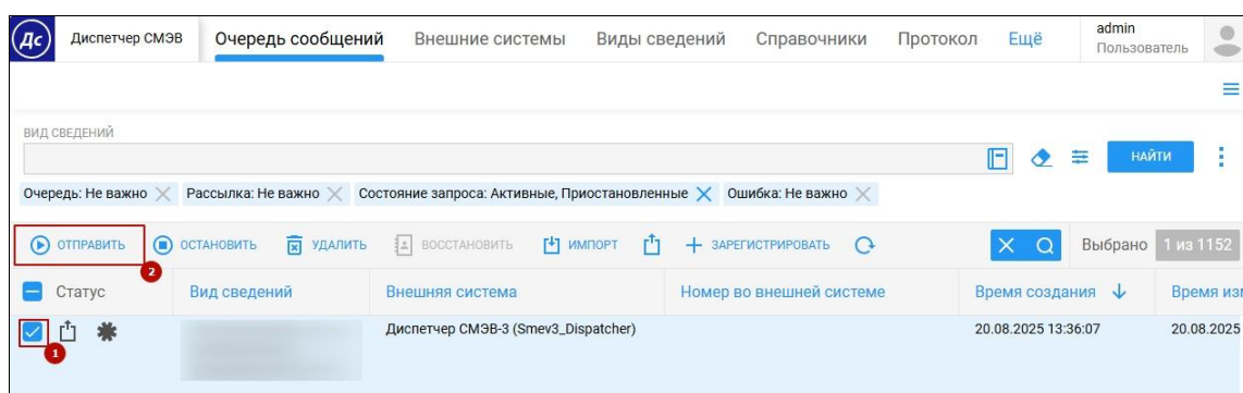
Рисунок 7. Отправка запроса
