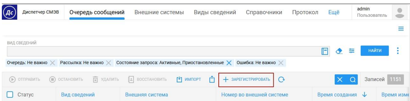
Рисунок 3. Регистрация запроса
