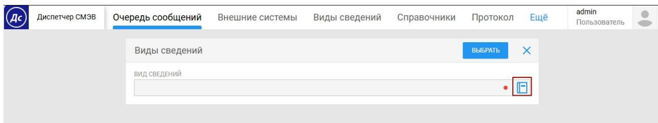
Рисунок 4. Выбор ВС
